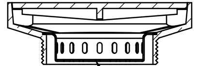
-80 SS BASKET (PN: 005270)
